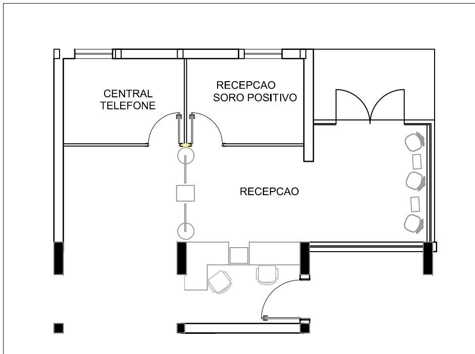
01 NOVO LAYOUT DE MOBILIÁRIO – RECEPCÃO S/ ESC.
